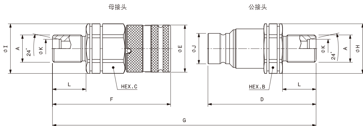
螺纹接口：外螺纹 L系列24° 锥隔板式 (ISO 8434-1& DIN 2353)
