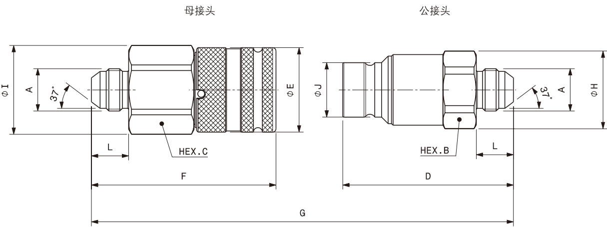
螺纹接口：外螺纹 JIC ( ISO 8434-2& SAE J514 )
