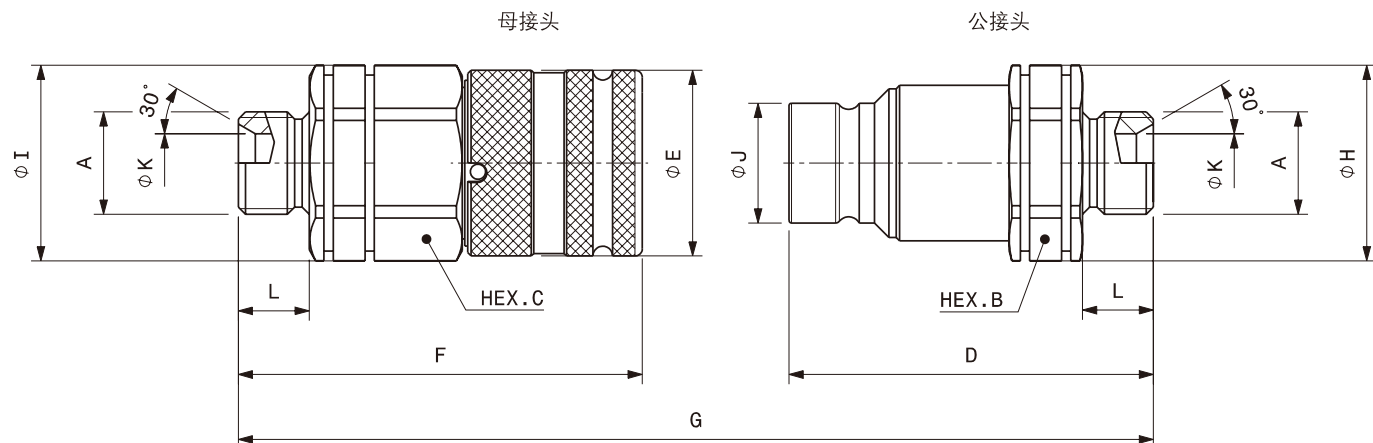
螺纹接口：外螺纹BSP ( ISO 8434-6 )
