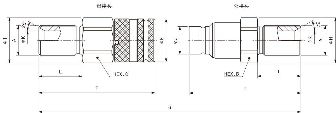
螺纹接口：外螺纹 BSP隔板式 ( ISO 8434-6 )
