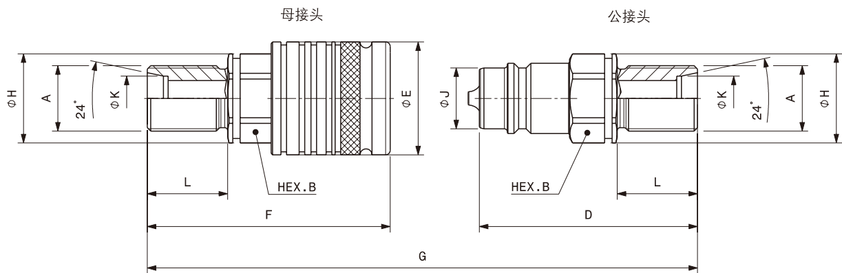
螺纹接口:公制外螺纹L系列-24° 锥隔板式 (ISO 8434-1 & DIN 2353)
