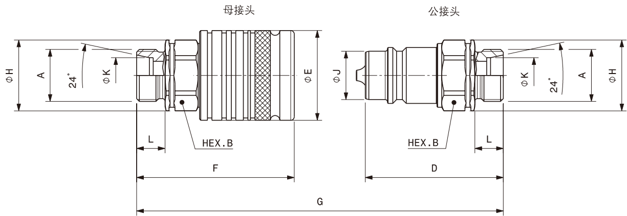
螺纹接口: 公制外螺纹L系列轻载-24° 锥 (ISO 8434-1 & DIN 2353)
