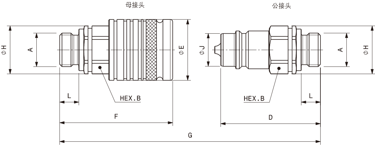
螺纹接口: 外螺纹 BSPP (DIN3852/A)
