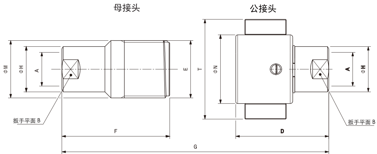
螺纹接口：内螺纹BSP (ISO 1179-1)
