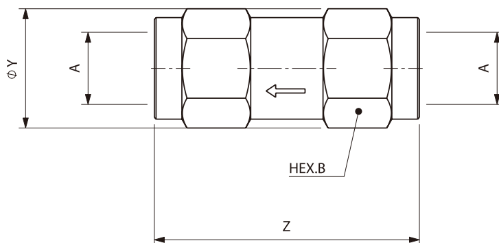
单向阀
